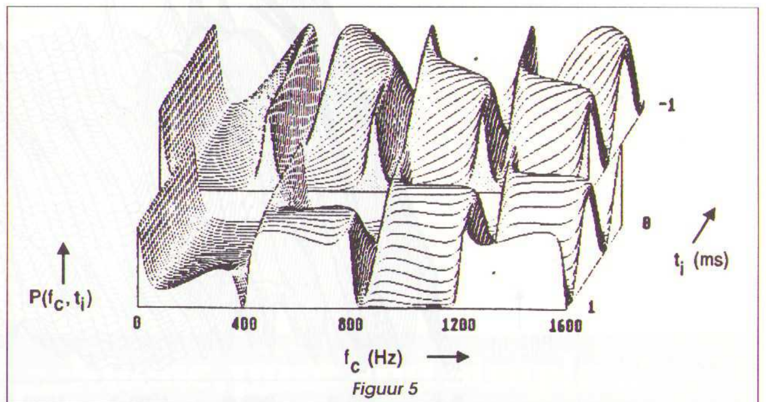
Figuur 5: Bij de aanbieding van de MPS-stimulus zoals geschetst in figuur 1A, ontstaat dit CAP. De grafiek is in het midden gesplitst om het centrale, harmonische, spectrum te laten zien.
